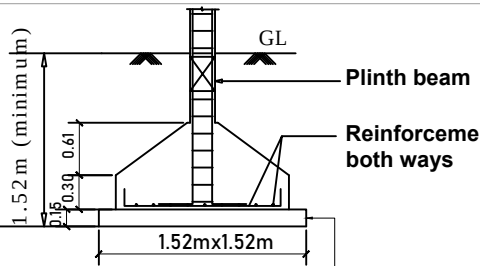
0.15m p.c.c 1:4:8 TYP.DET.COLUMN FOOTING
