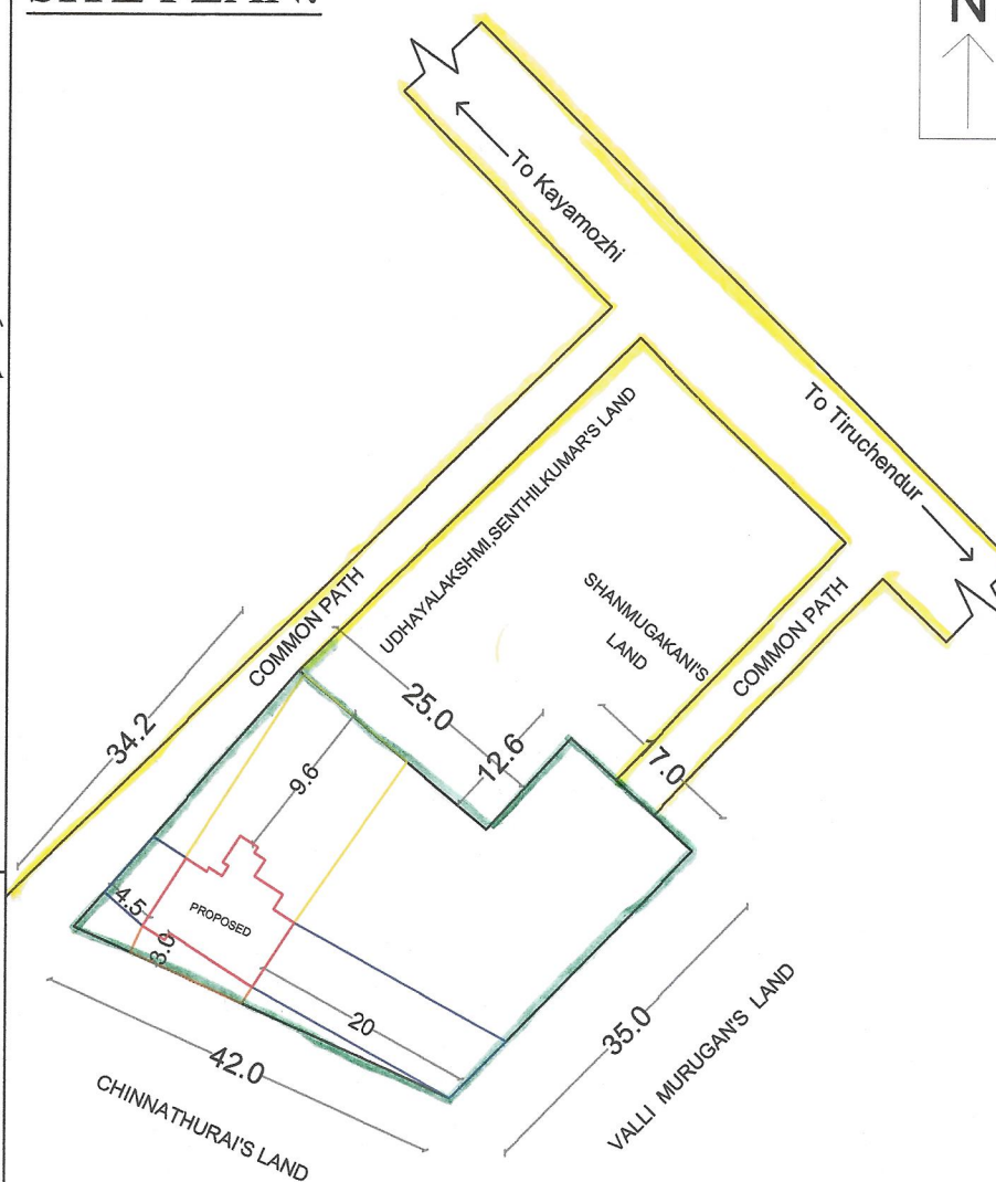
SITE PLAN:
