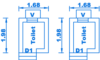
TOILET PLAN
