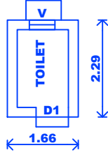
TOILET PLAN
