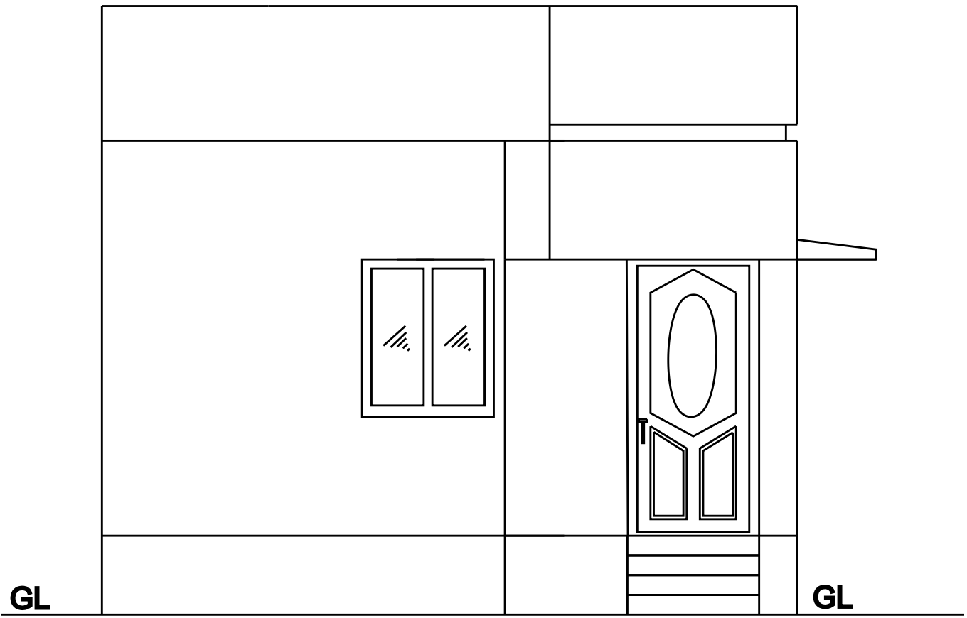
ELEVATION
