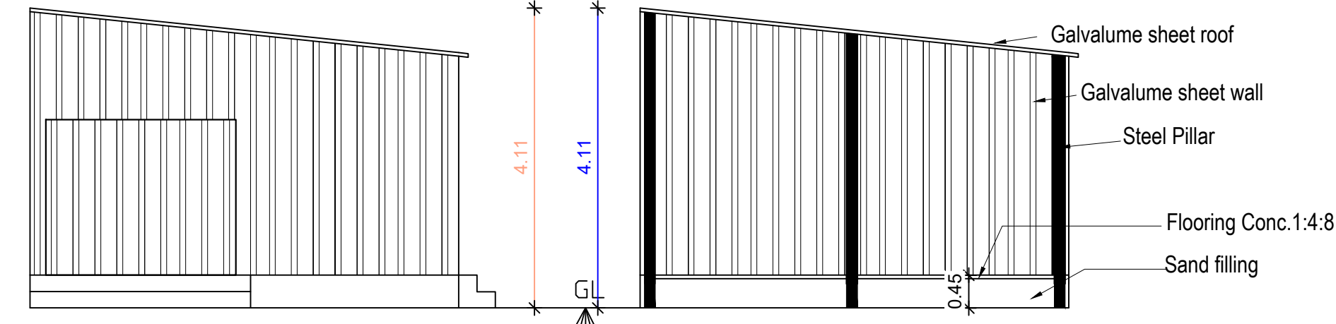
ELEVATION
