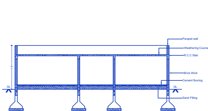
SECTION-A
