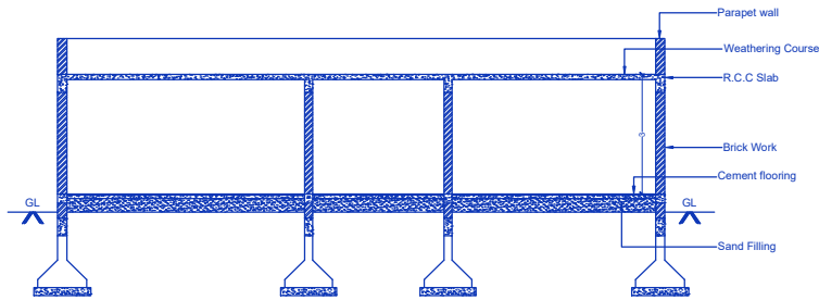
SECTION-A
