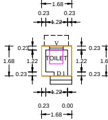
TOILET PLAN
