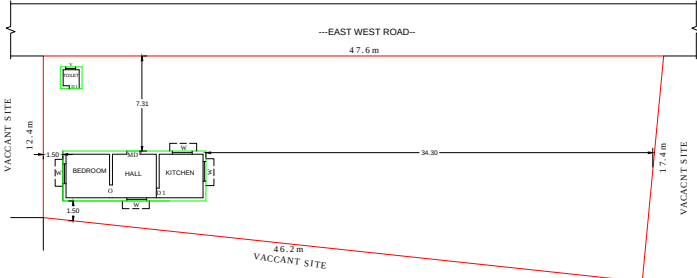
SITE PLAN (SCALE : 1:200)
