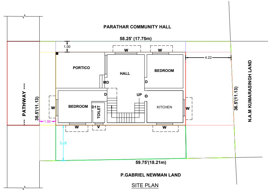
( SCALE : - 1:100 )
