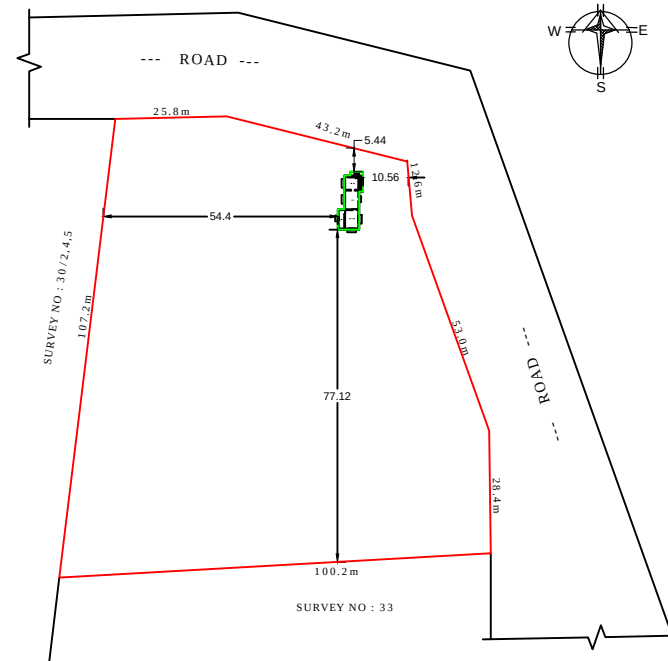
SITE PLAN (SCALE : - 1:800)
