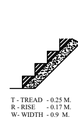
STAIRCASE DETAILS - N.T.S
