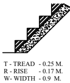
STAIRCASE DETAILS - N.T.S
