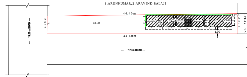
SITE PLAN (SCALE : - 1:200)
