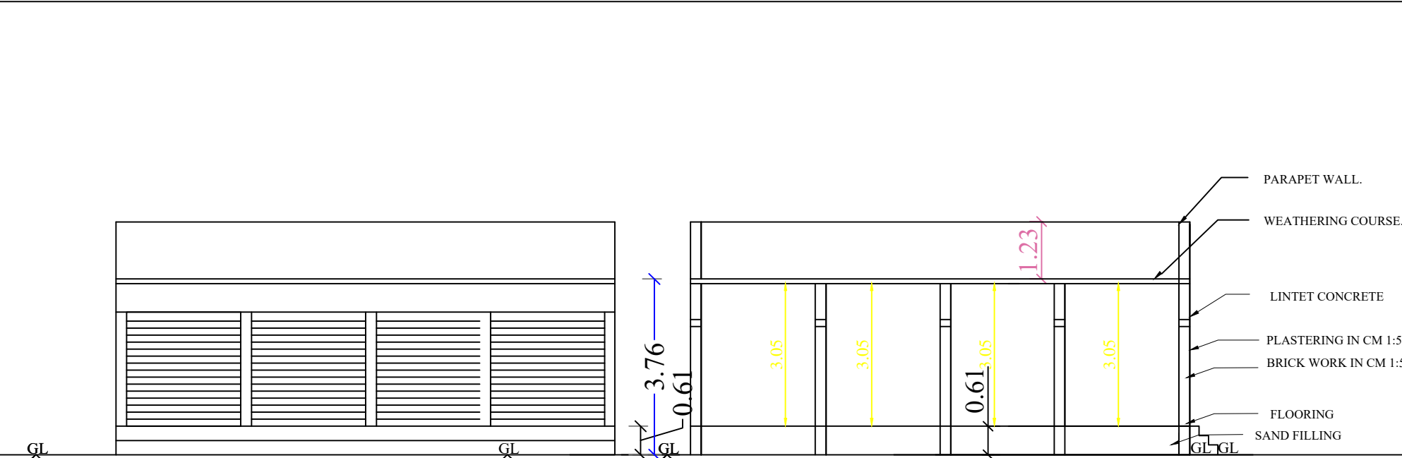
ELEVATION
