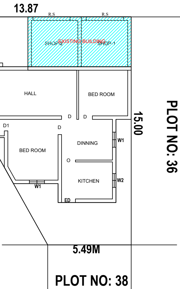
SITE PLAN ( SCALE 1:150)
