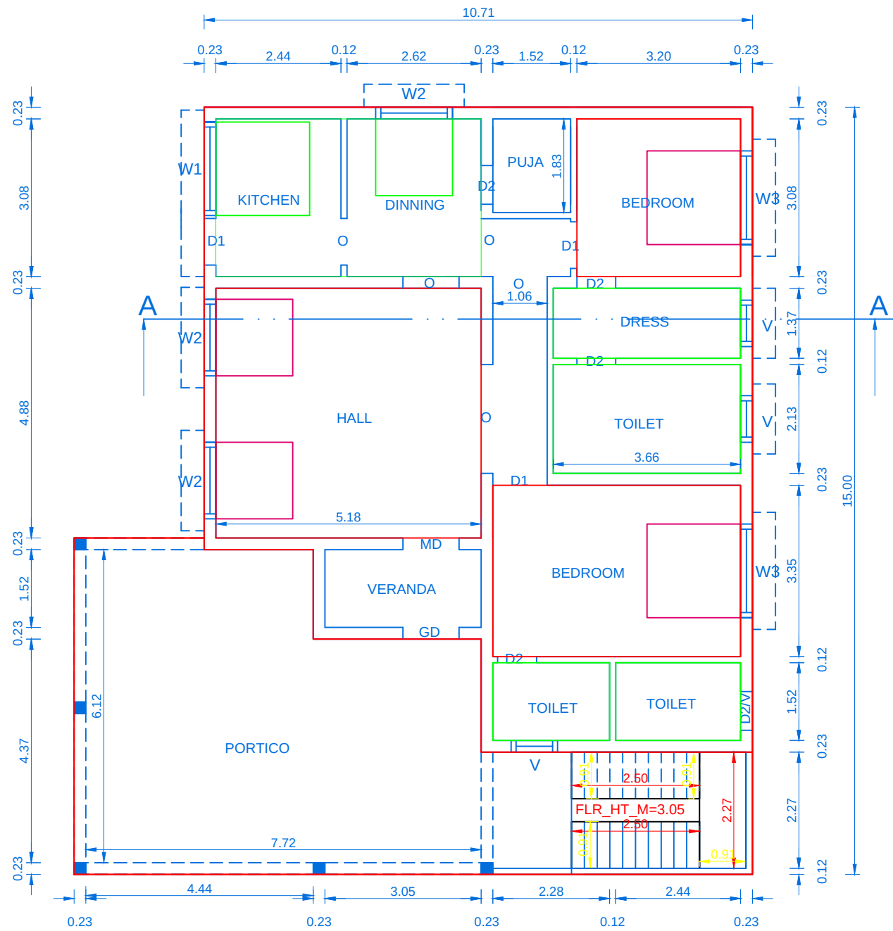
DR PLAN
