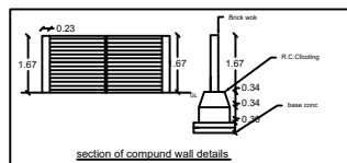
ELEVATION
