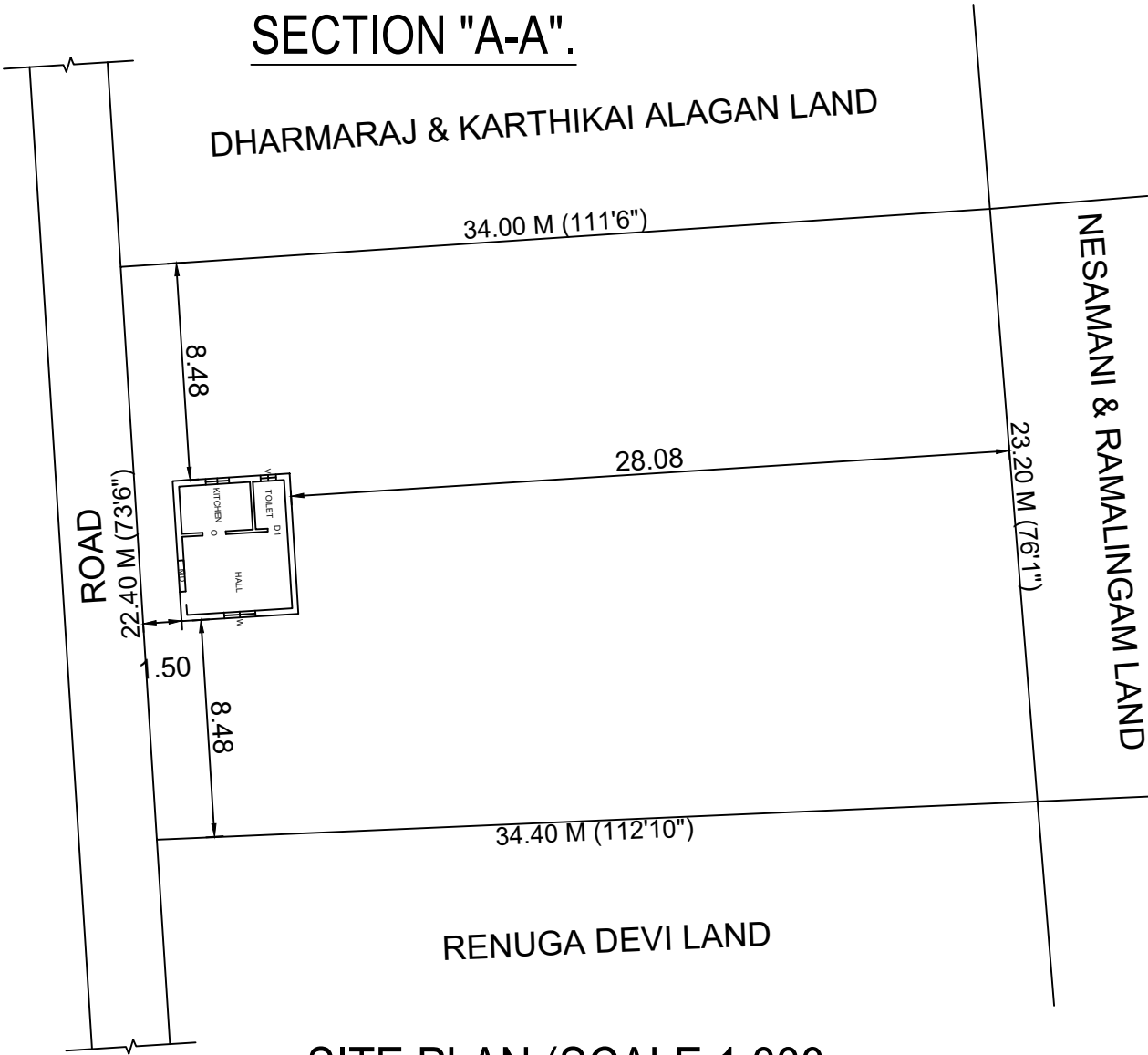
SITE PLAN (SCALE 1:333)
