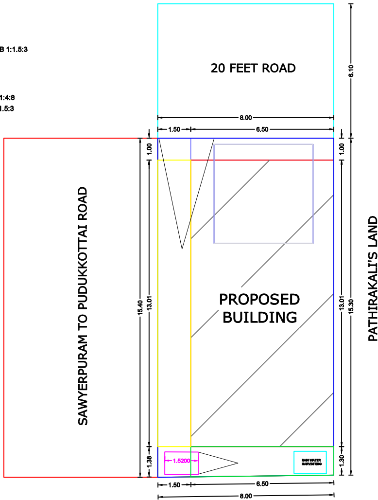
SITE PLAN: 1:100
