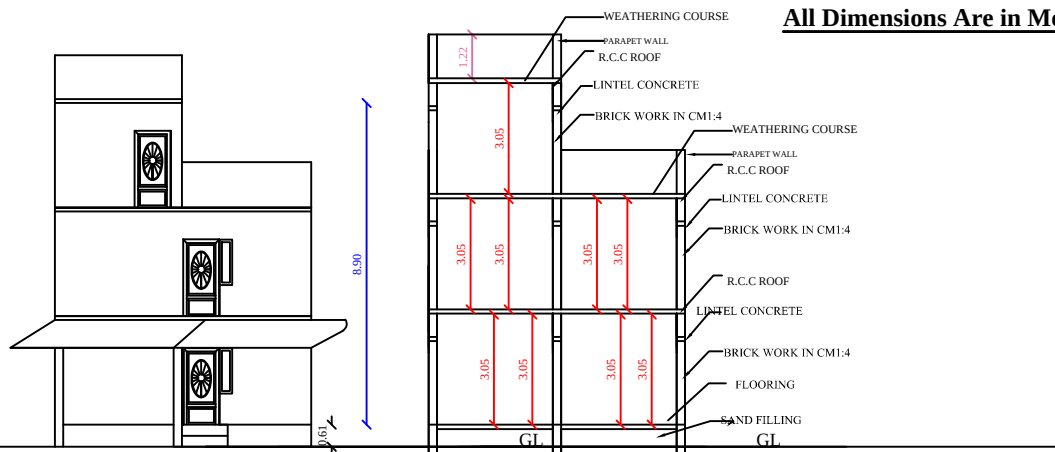
ELEVATION
