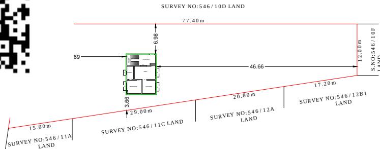
SITE PLAN SCALE 1:400
