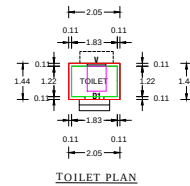
TOILET PLAN
