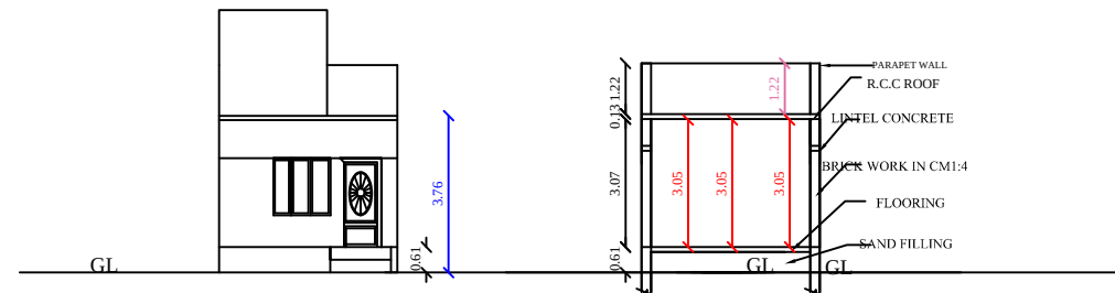
ELEVATION
