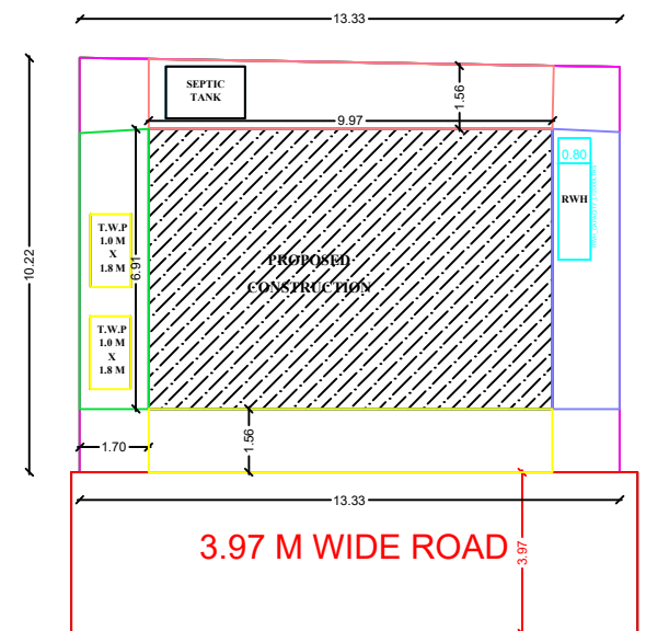
SITE PLAN SCALE : 1"= 8' OR [1 : 100]
