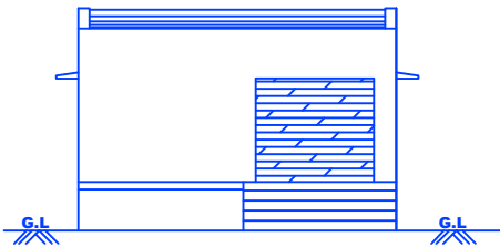
ELEVATION - AA
