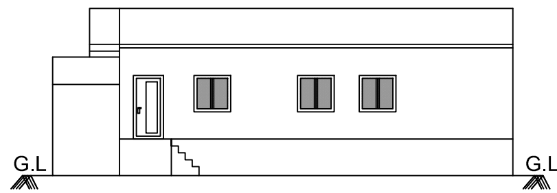
ELEVATION
