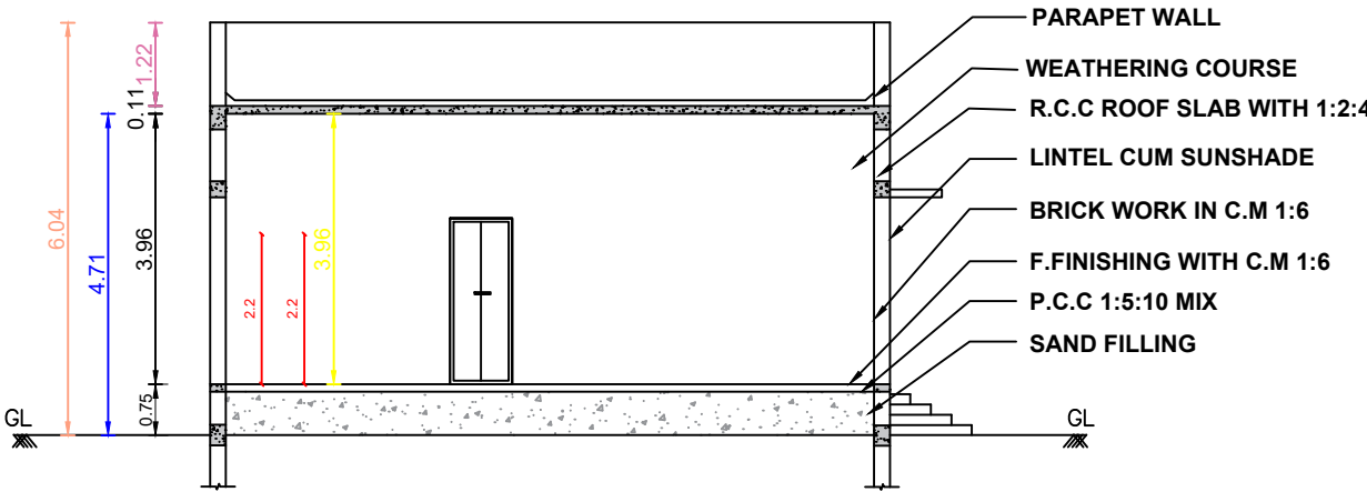
SECTION "A-A".
