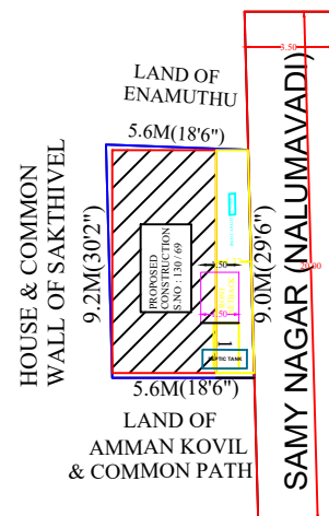
STE PLAN
