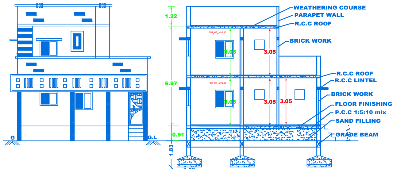
ELEVATION
