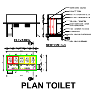
PLAN TOILET
