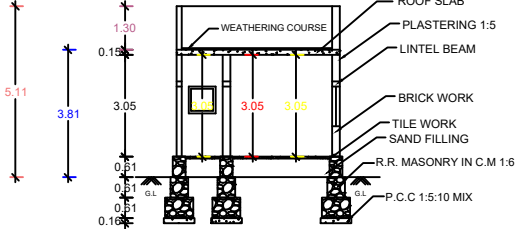
SECTION A-B
