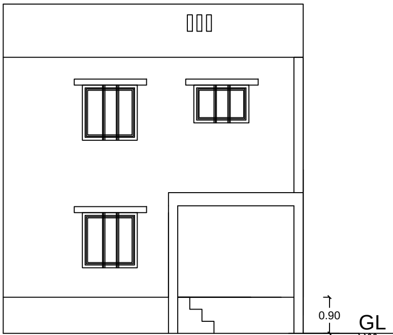
ELEVATION
