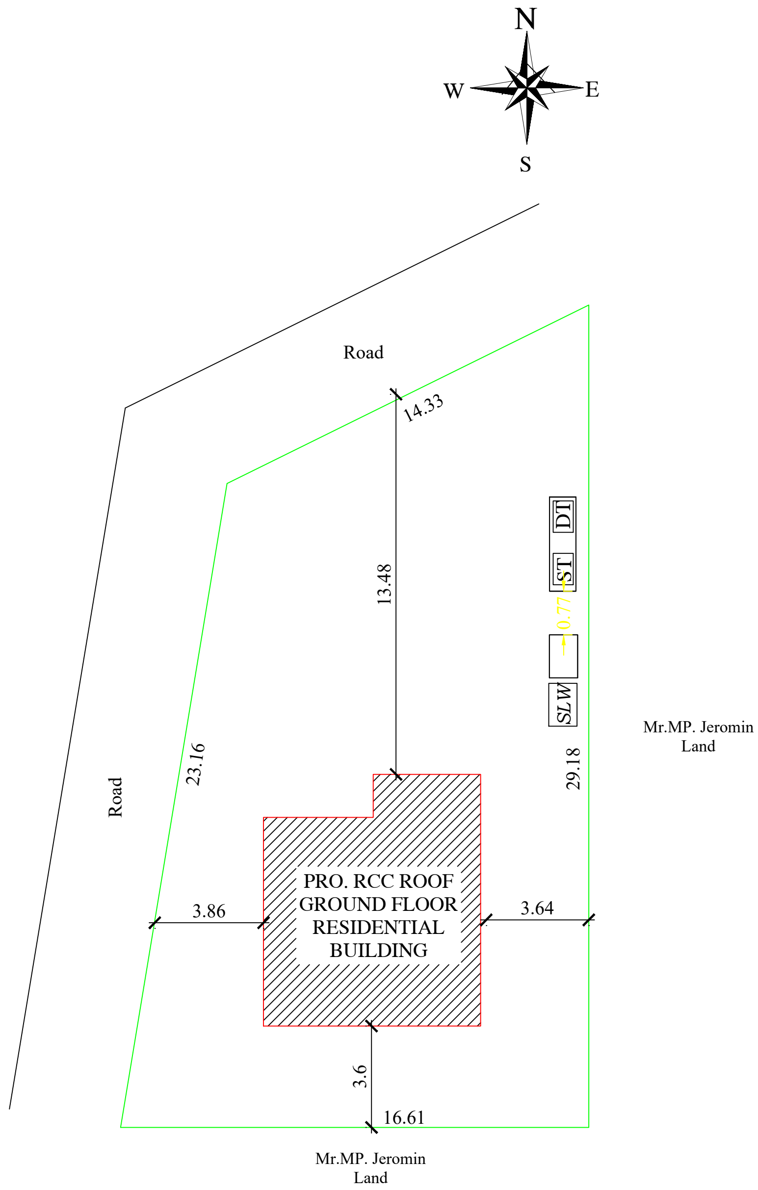
SITE PLAN - 1:200
