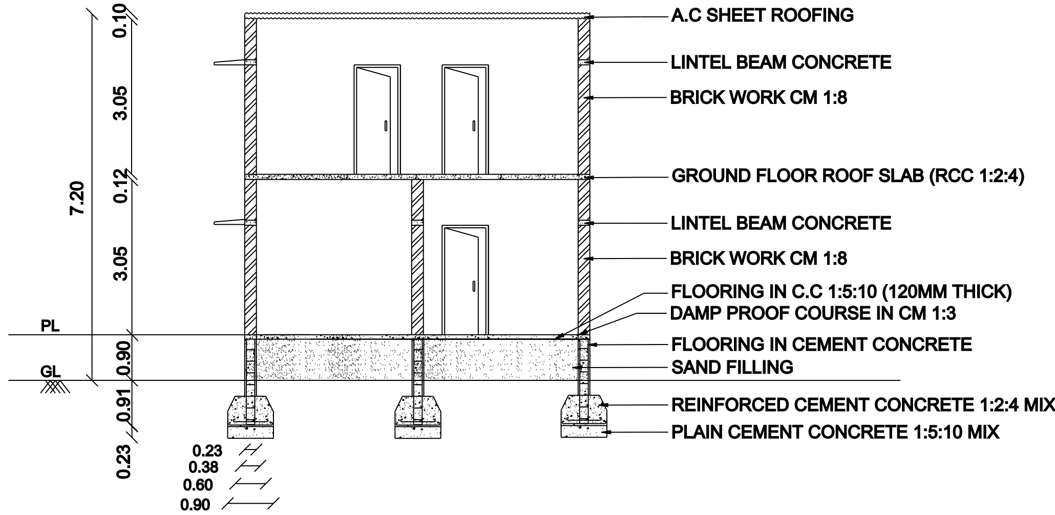
SECTION A-B
