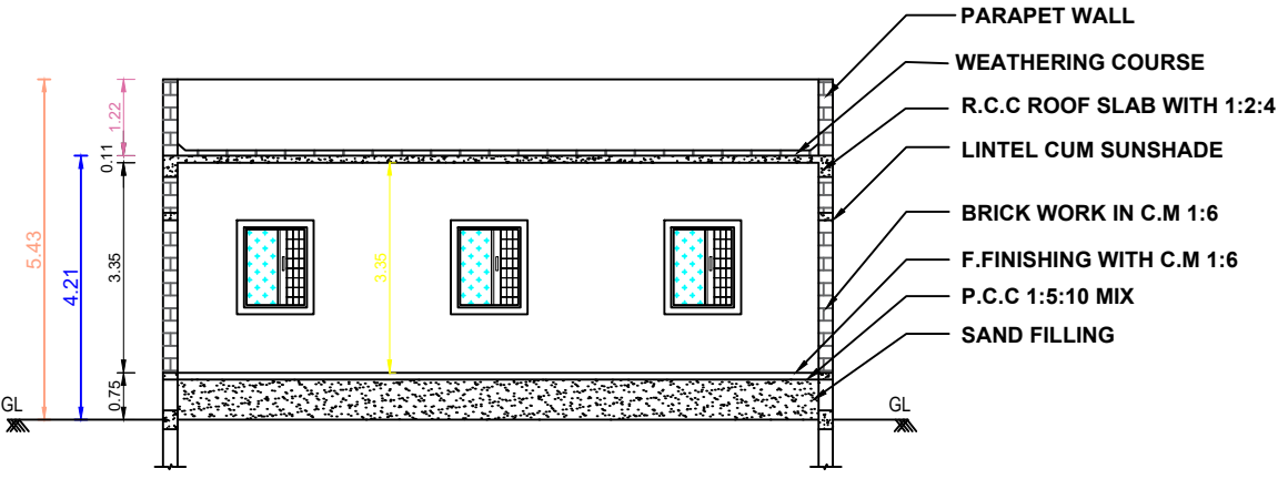
SECTION (A-A)
