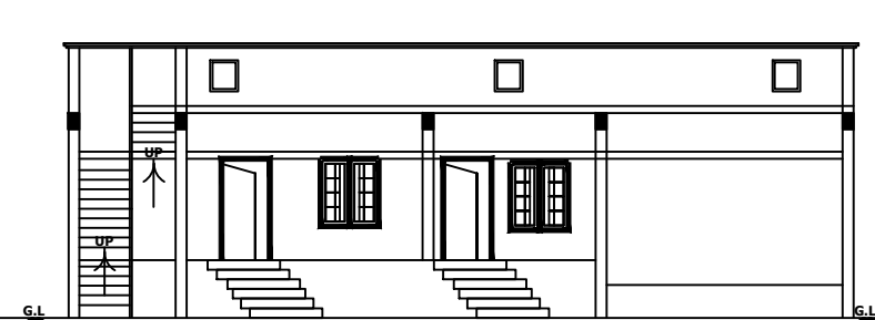
ELEVATION
