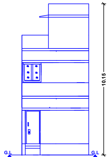
ELEVATION
