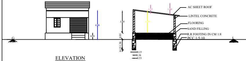
ELEVATION
