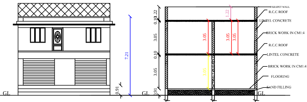
ELEVATION
