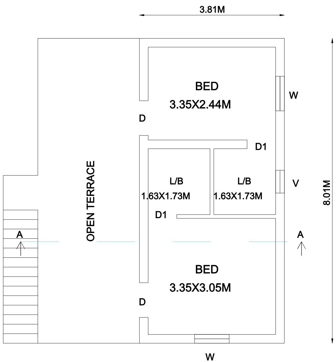
PRO. F.F. PLAN
