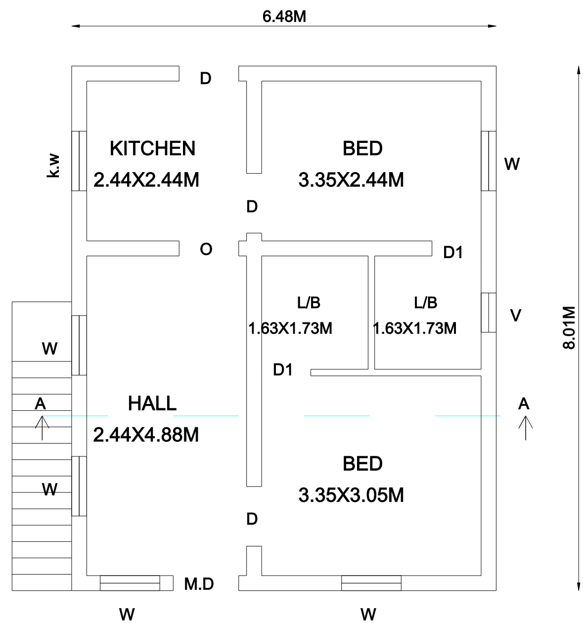
PRO. G.F. PLAN
