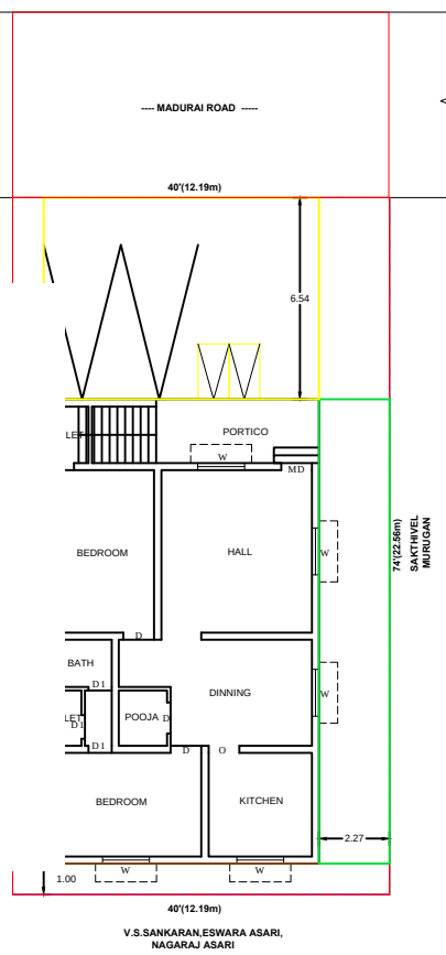
SITE PLAN (SCALE : - 1:100 )
