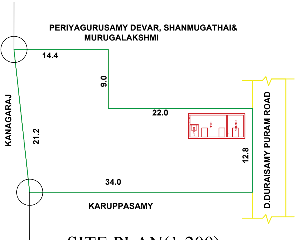
SITE PLAN(1:200)
