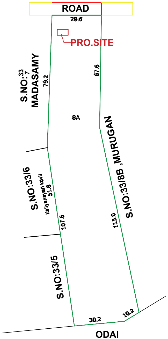
SITE PLAN(1:500)
