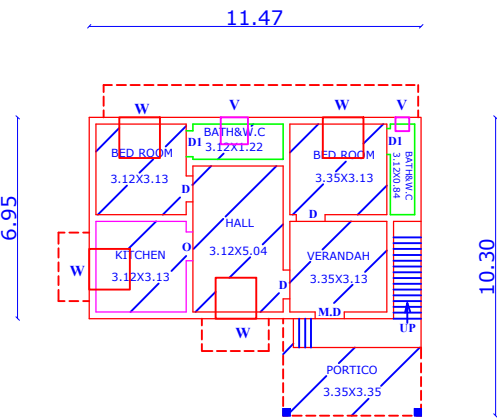
EXG-G.F.HOUSE PLAN
