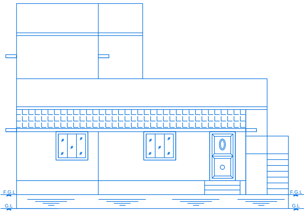
ELEVATION
