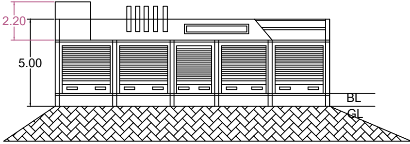
ELEVATION
