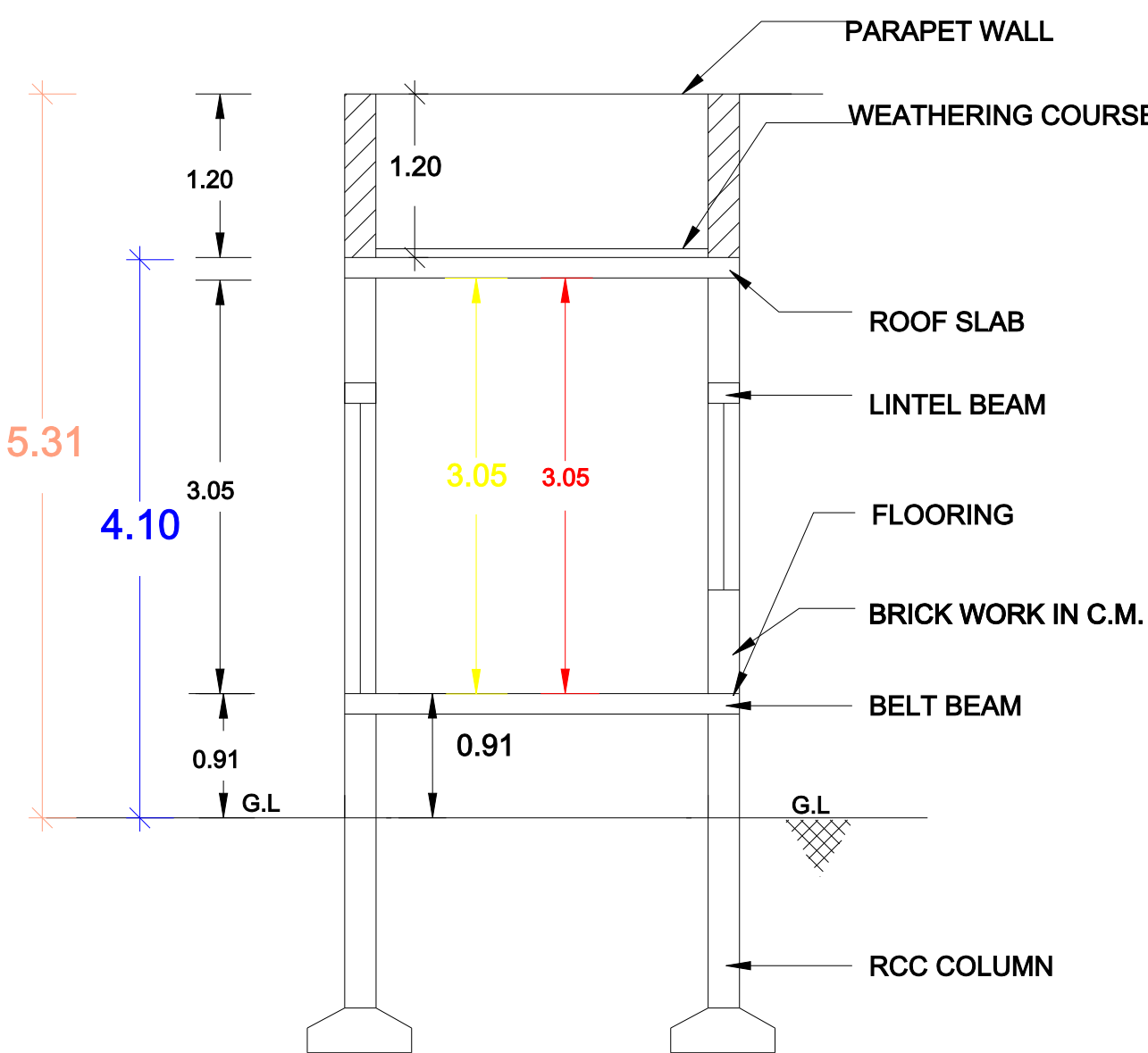
SECTION A-A
