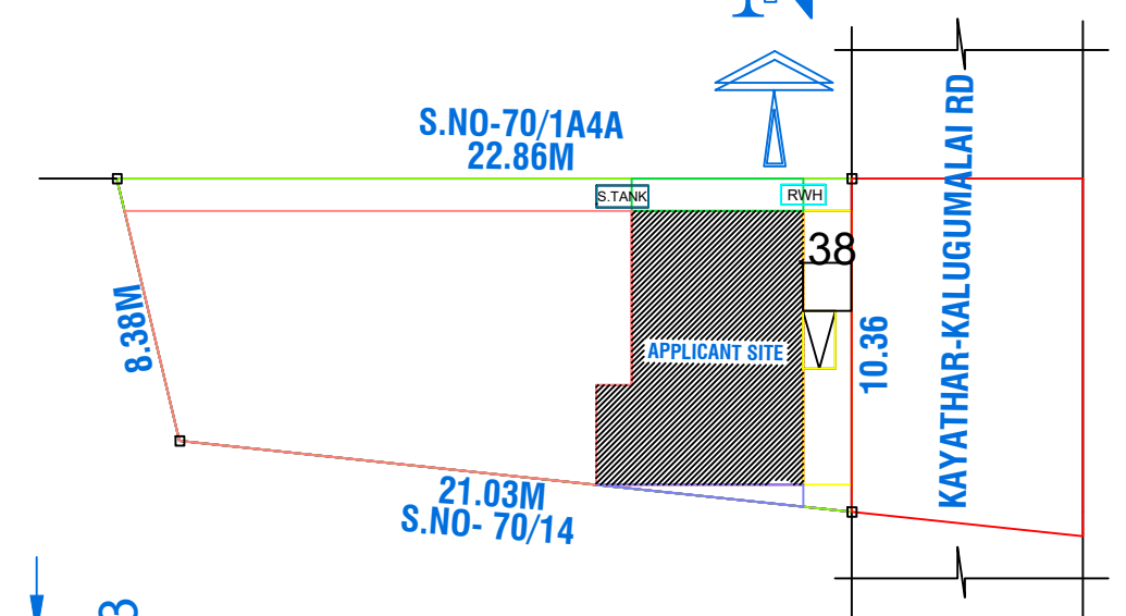
SITE PLAN(1:400)
