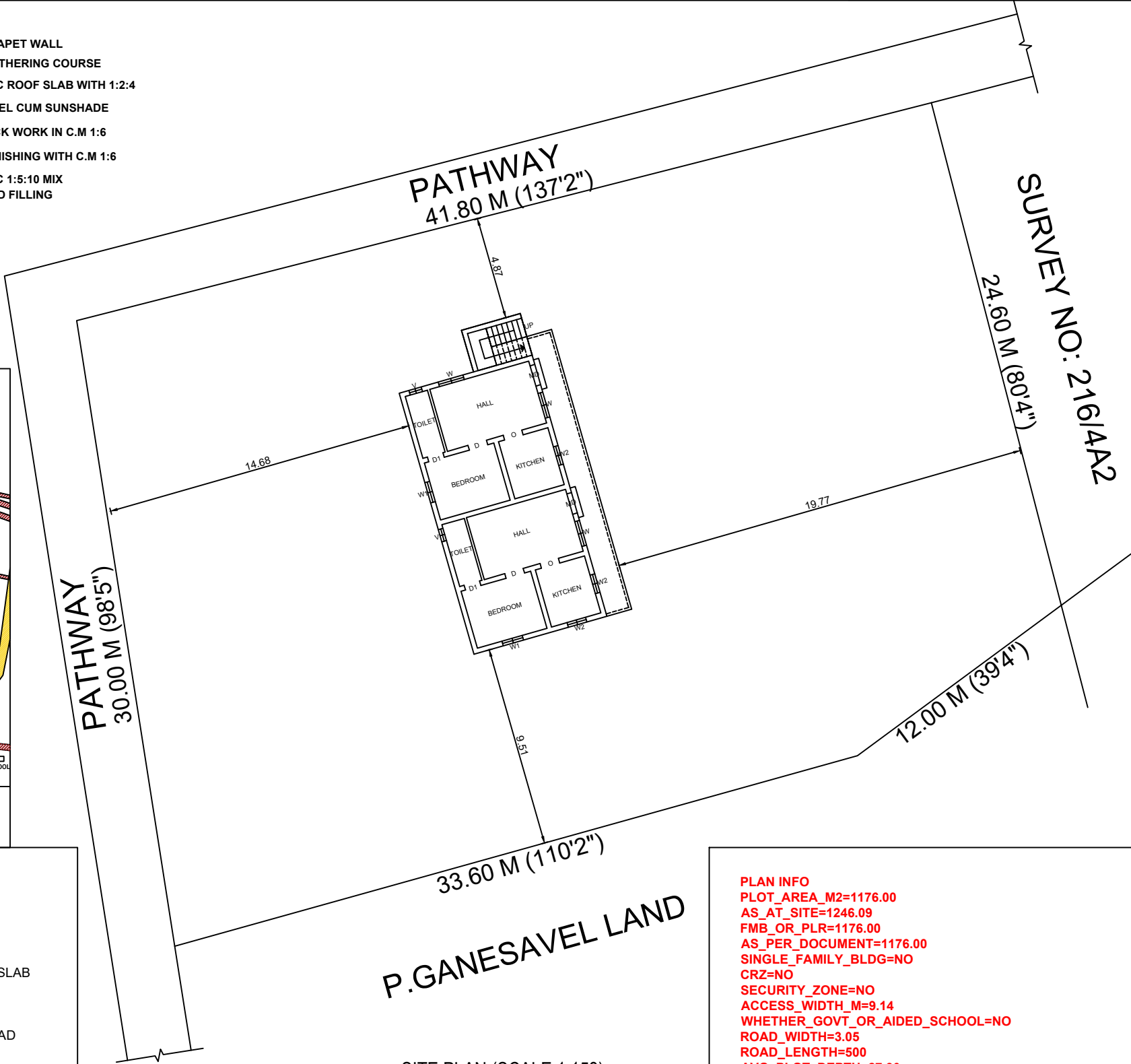
SITE PLAN (SCALE 1:153)
